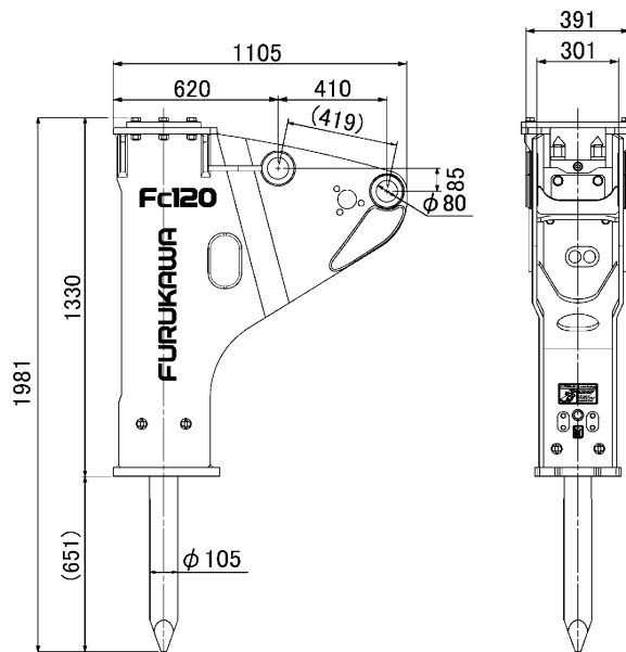
ピン間距離: 419mm
