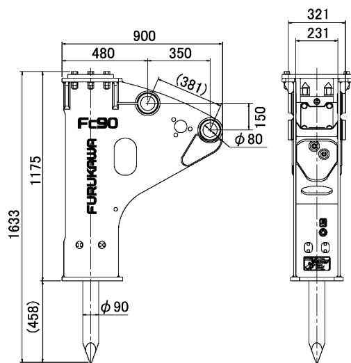
ピン間距離: 381mm
