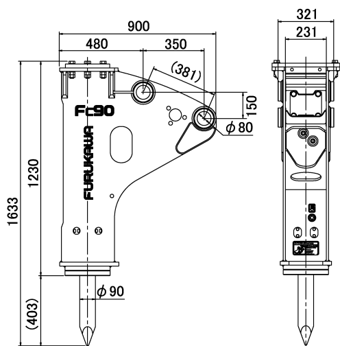
ピン間距離: 381mm
