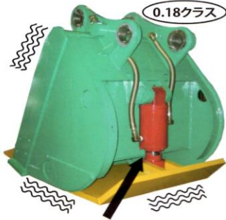
油圧振動装置 <ウエダターボジャック>
